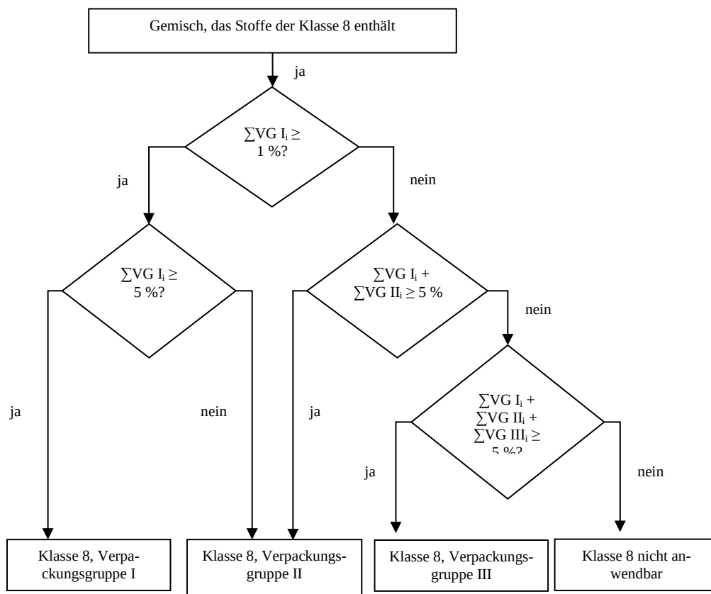
Abbildung 2.2.8.1.6.3: Berechnungsmethode
